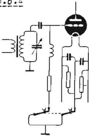
Sleutelen, tegeliktijd in roostercircuit en anodekring.
